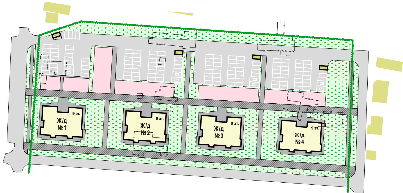
План озеленения территории М 1 : 1 500
