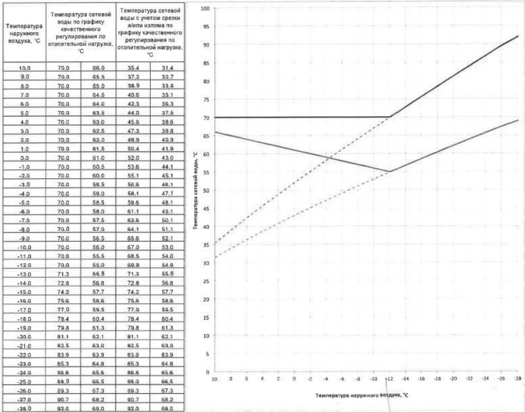
Температурный график работы тепловой сети от теплоисточников филиала "Мордовский" ПАО "Т Плюс": котельные Баниа №3 по ул.Кутузова, 2Б; Кирзавод по ул.Осипенко, 8; пос. Горяиновка (ОПХ 1 мая) по ул.Молодежная, 13А; пос. Зыково по ул.Советская, 124 Е на отопительный сезон 2023-2024 г.г.
