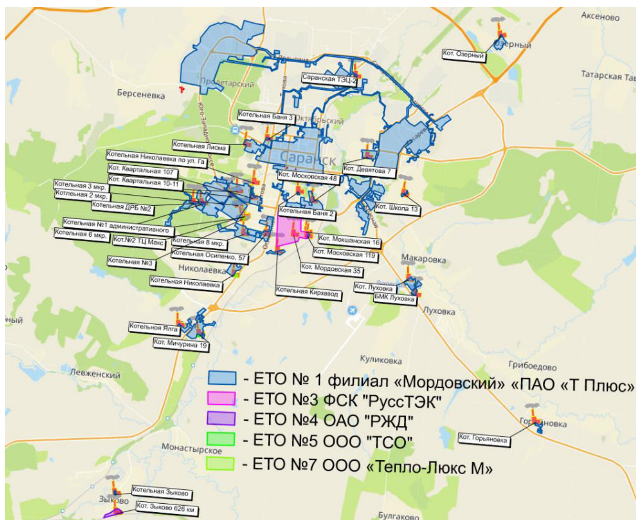
Рисунок 28. Границы зон деятельности единой теплоснабжающей организации
