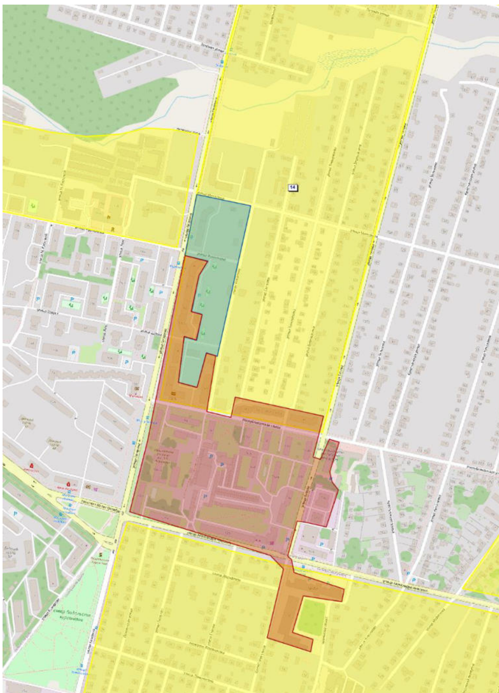
Рисунок 16. Существующая (выделена красным) и перспективная (выделена синим) зоны действия котельной кв. 107 после подключения новых площадок застройки (выделены желтым)
